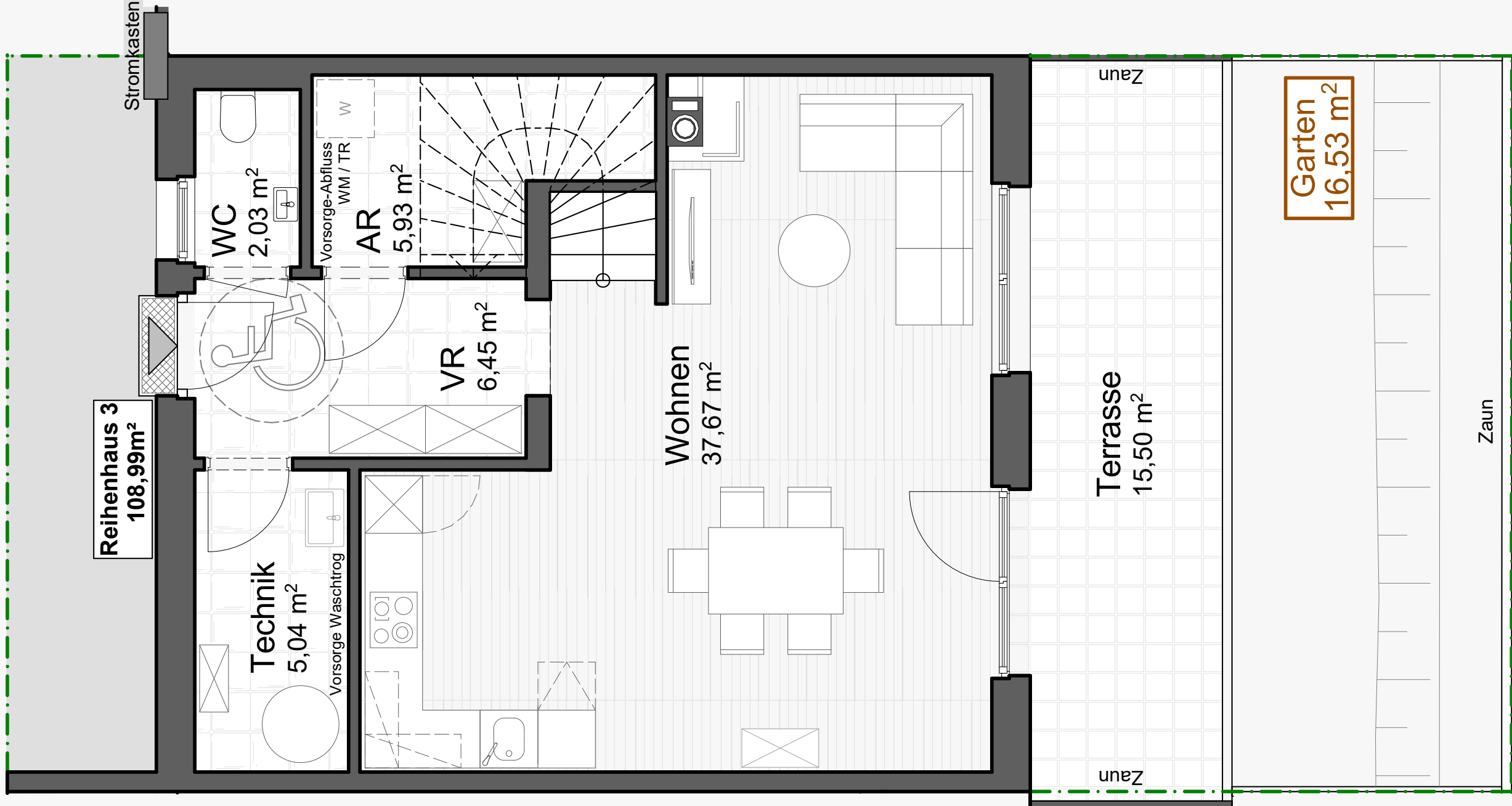
Erdgeschoss
