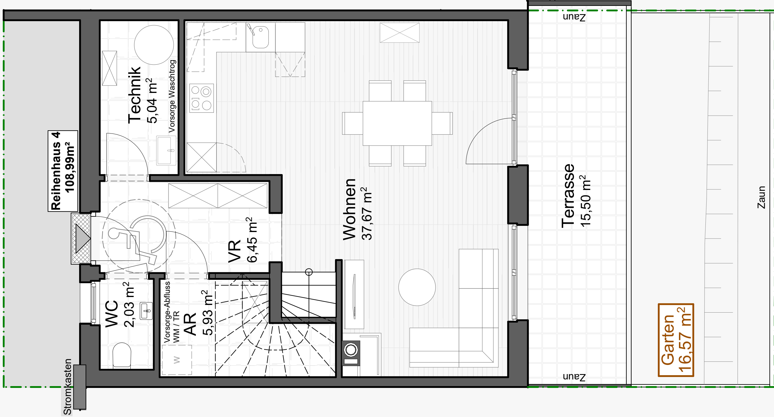
Erdgeschoss
